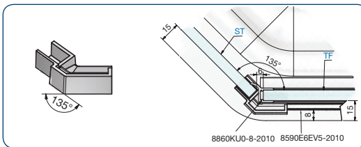
Art.-Nr. 8596KU7-L Fünfeckverbinder links-Türband links
