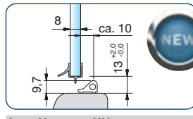
Art.-Nr. 8879KU0-8-2010 für 8 mm Glas in Verbindung mit dem Schwallenschutzprofil (Art.-Nr. 8535E6EV5)
