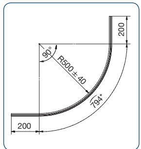
Art.-Nr. 8867KU0-8-R500 gebogen für Wannensradius R500 - 550 für 6 und 8 mm Glas Abwicklung = 1194 mm
