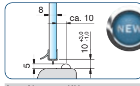
Art.-Nr. 8879KU0-8-2010 für 8 mm Glas in Verbindung mit dem Acrylhalbrundstab (Art.-Nr. 8538KU5, Radius = 5 mm)
