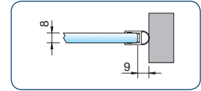
Art.-Nr. 8861KU7-8-2010 Dichtprofil für den seitlichen Wand- anschluss 90° (Beslagseite) für 6 und 8 mm Glas für ein ein- und beidseitig zu öffnendes Duschtürband
