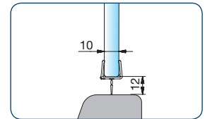
Art.-Nr. 8876KU0-12-2500 für 10 und 12 mm Glas
