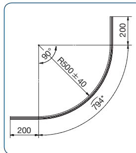
Art.-Nr. 8881E6/500 Art.-Nr. 8882E6/500 Art.-Nr. 8881E0/14-R500 Art.-Nr. 8882E0/14-R500
