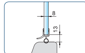
Art.-Nr. 8867KU0-8-R500 gebogen für Wannensradius R500 - 550 für 6 und 8 mm Glas Abwicklung = 1194 mm
